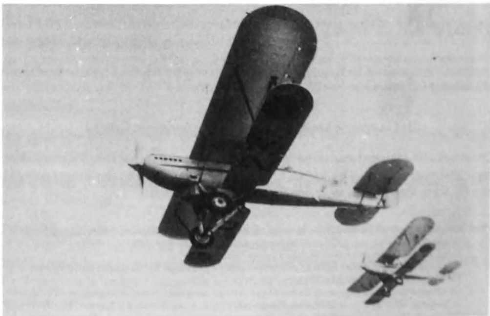
Fairey Fox met Rolls-Royce Kestrel-motor; type II, "0.23".
